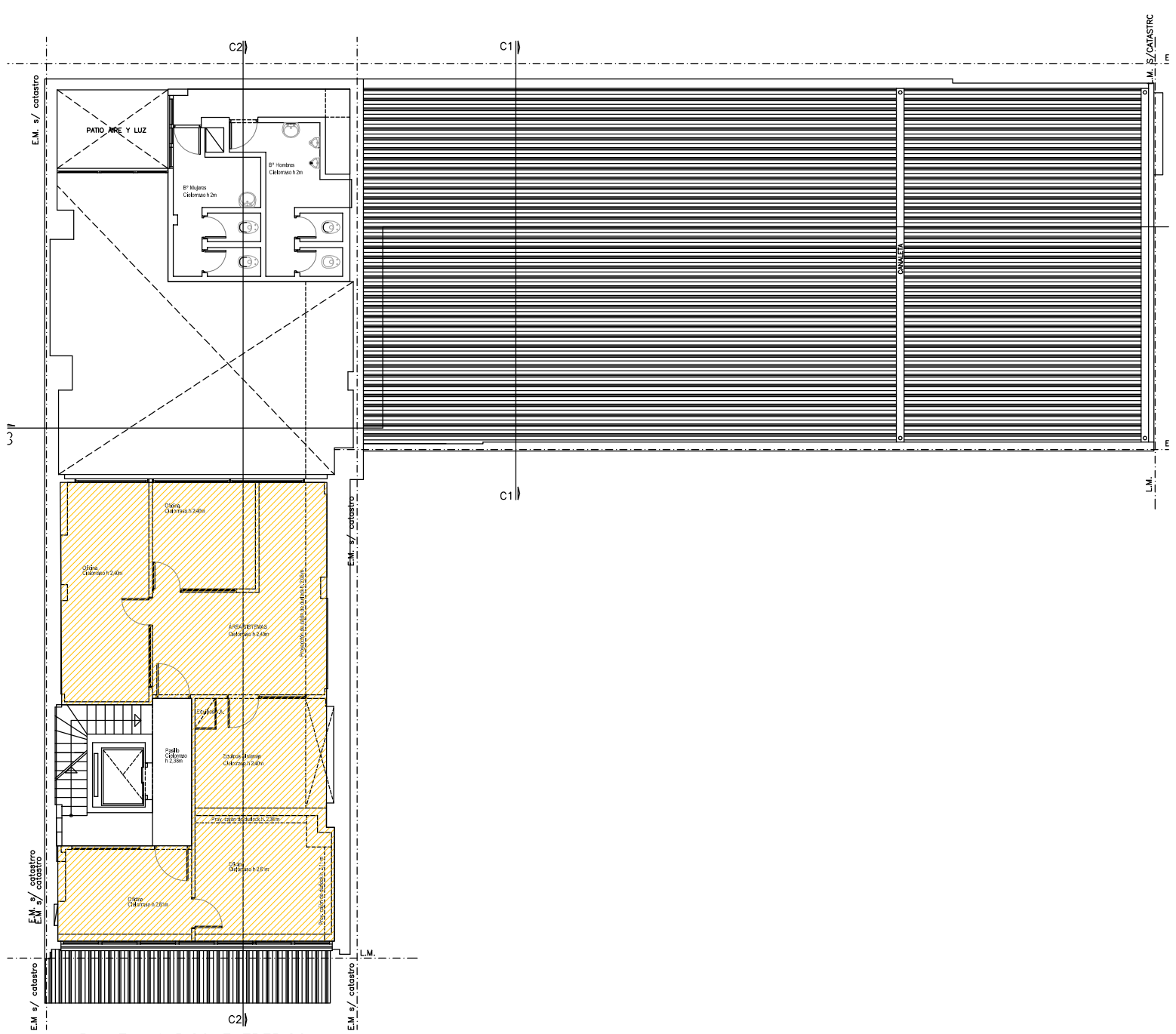
PLANTA 1° PISO ENTREPISO
