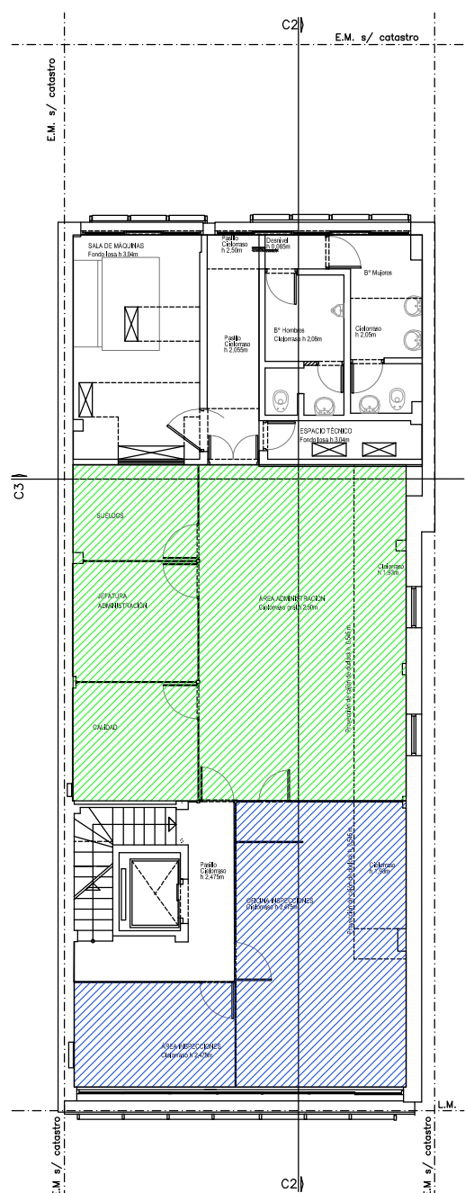
PLANTA 3º PISO
