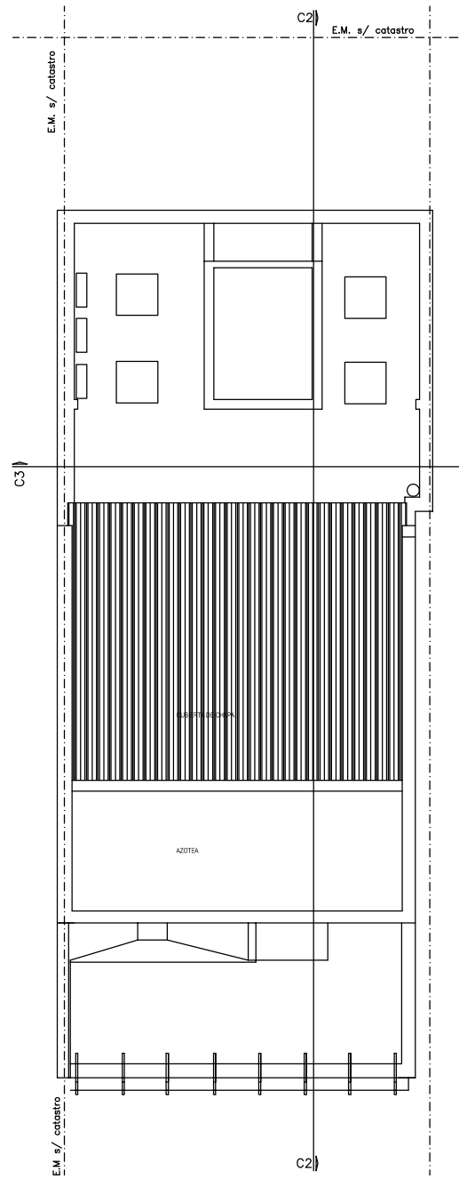
PLANTA DE TECHOS
