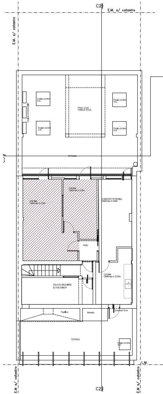
PLANTA 6° PISO
